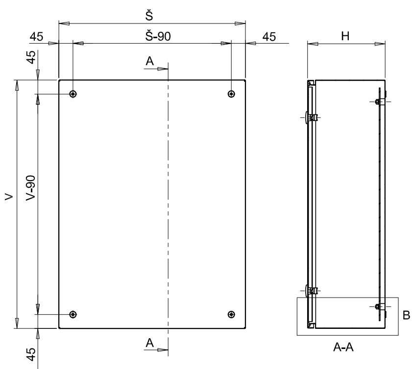
Rozteče upevňovacích otvorů ASTRA
