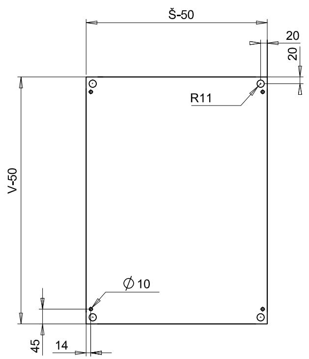
Montážní panel skříně ASTRA
