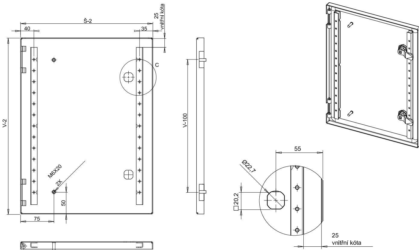
Detail dveří skříně ASTRA (jazýčkový zámek)
