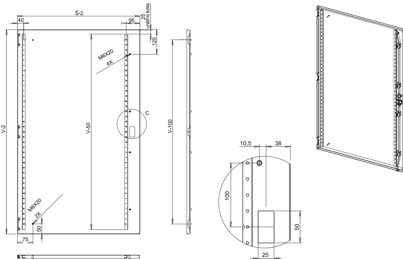
Detail dveří skříně ASTRA (rozvorový zámek)
